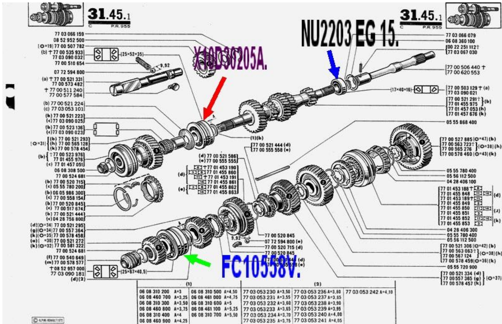
Roulement des BV 365 des Alpines A310 4 cylindres.....
