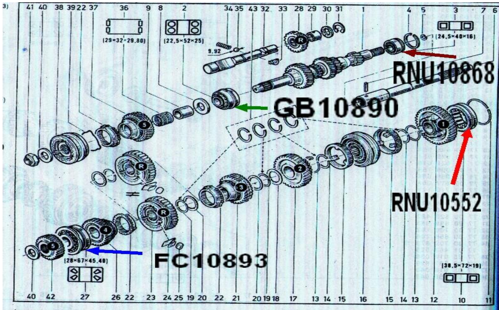
Roulements des 2 arbres de BV NG5 Renault 5 Alpine turbo.....
