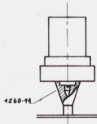
Montage d'allumeur pour GS citroën
