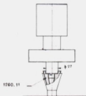
Montage d'allumeur modèle à queue de 27 mm, français (suivant BNA.9) et étranger, Toc rapporté au flottant.
