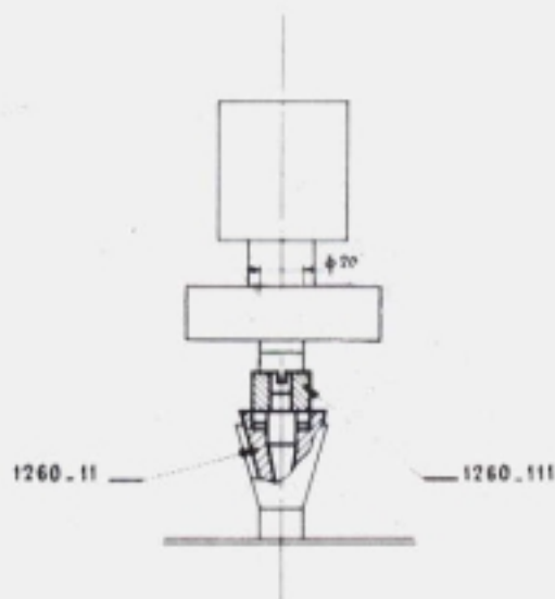
Montage d'allumeur modèle à queue de 20 mm sur véhicule Panhard.
