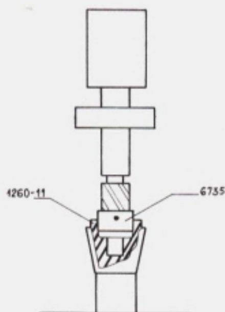
Montage d'allumeur à queue Pour SM
